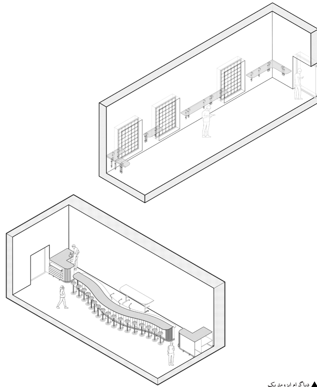
▲ دیاگرام ایزومتریک
